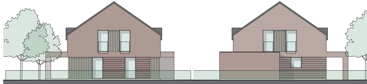
SE Side Elevation 1:75 @ a1
